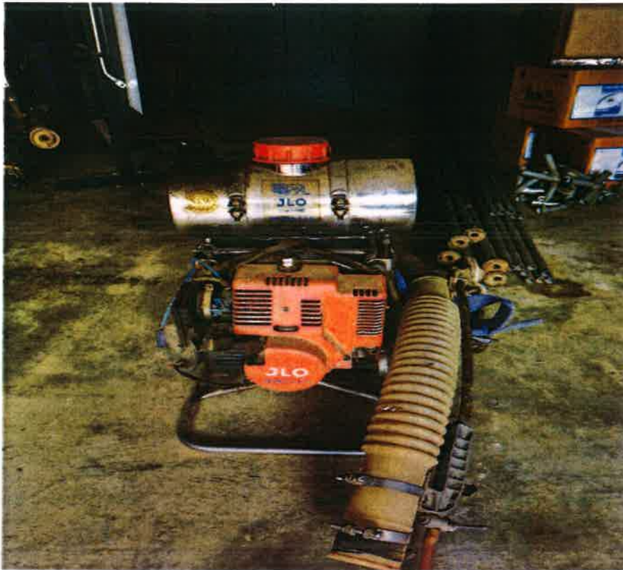
เครื่องพ่นละอองฝอย ULV รหัส ๖๒๕-๕๕-๐๐๐๒
